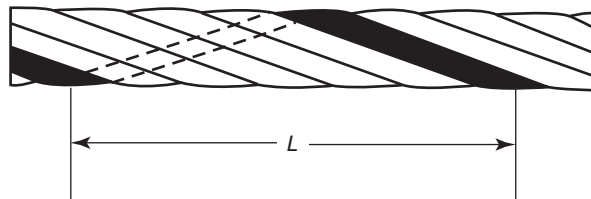
Fig. 1.3.3.2.1-1 Strand Lay Length
