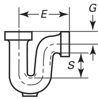
P-Trap
