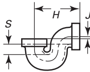
Bath P-Trap
