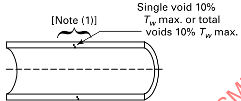
(d) Acceptable Voids (Microbubbles) in Melt Zone
