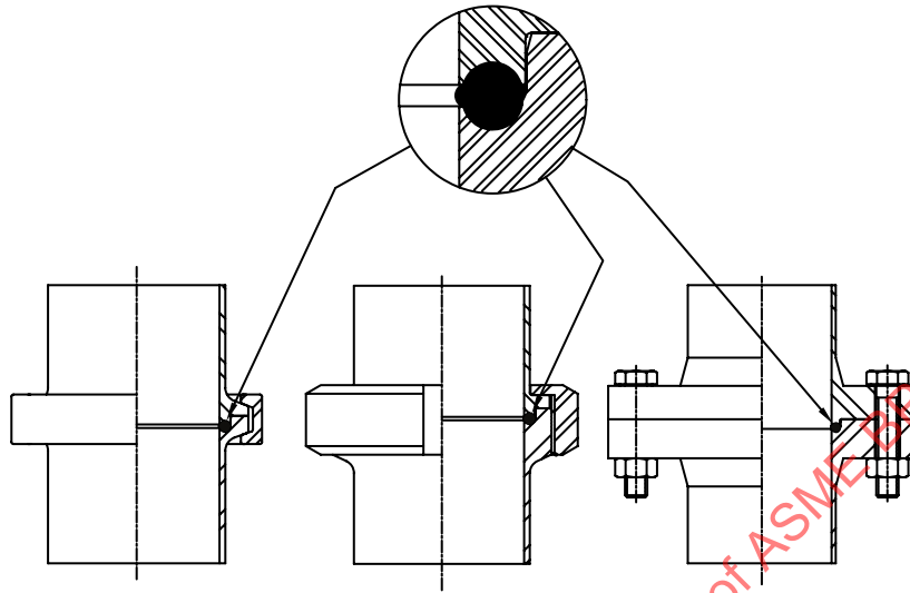
Figure MC-2.2.2-3 Hygienic Union per DIN 11864
