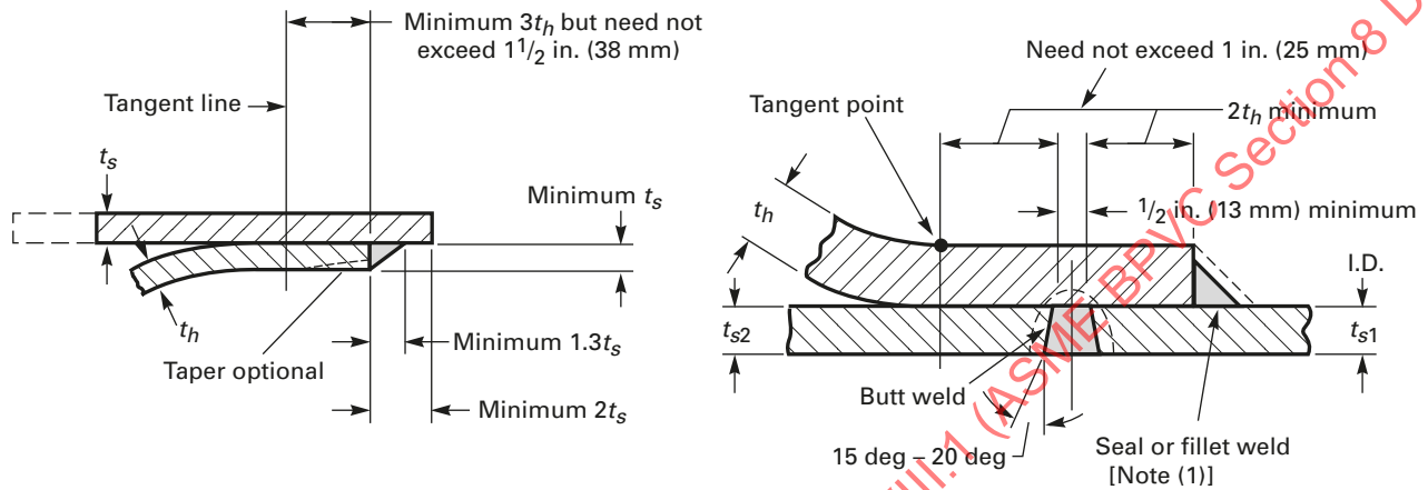
(d) Single Fillet Lap Weld
