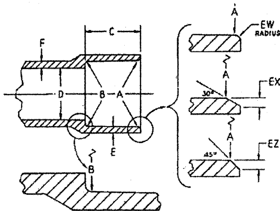
FIG. 1 Socket Dimension Symbols per D2749
