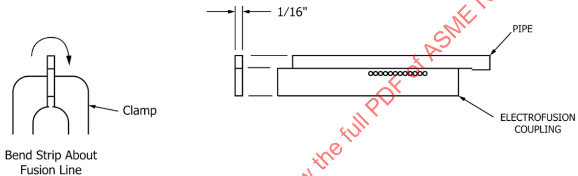
FIG. 13 Strip for FET Bend Test
