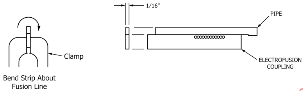
FIG. 8 Strip for FET Bend Test
