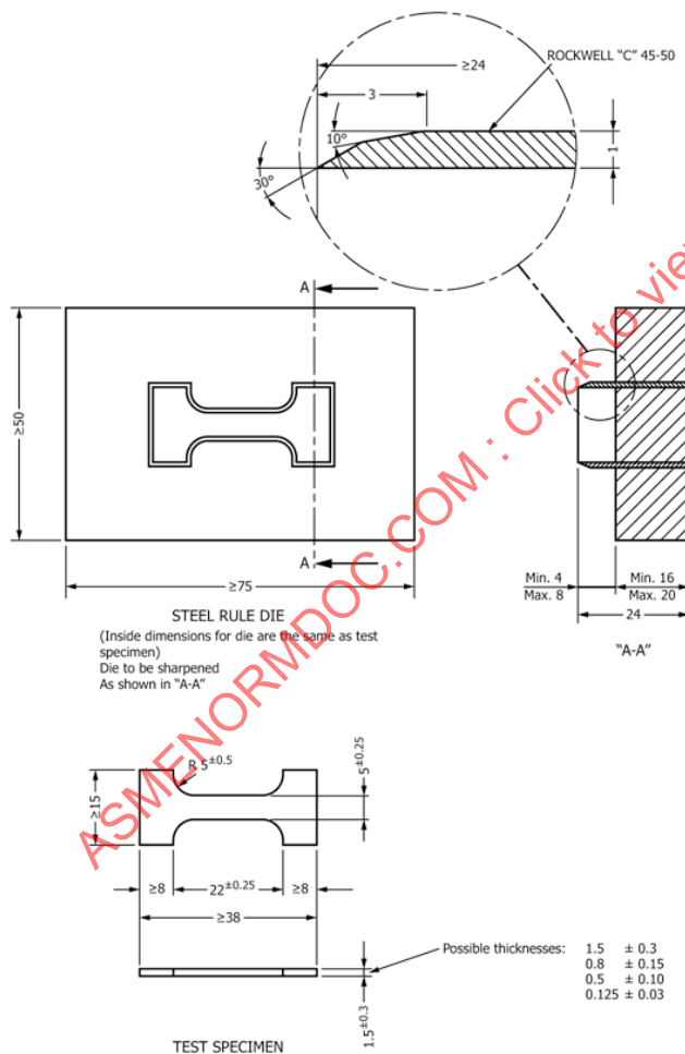
FIG. 8 Microtensile Die
