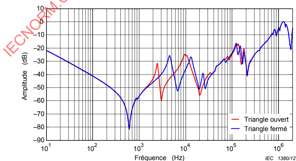
Figure B.7 – Effet d'une connexion en triangle tertiaire sur la réponse en fréquence d'un enroulement série
