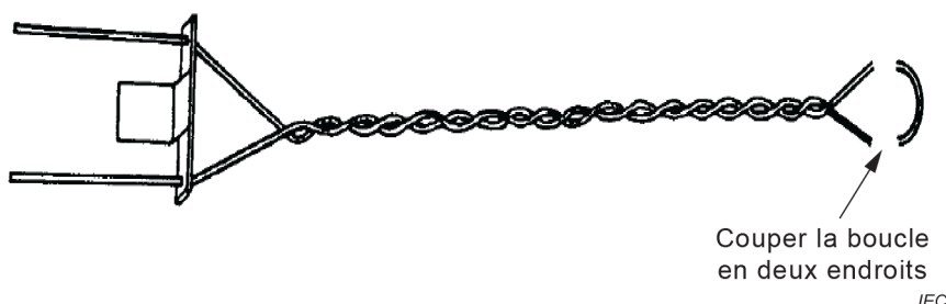
Figure 5 – Éprouvette réalisée, boucle coupée
