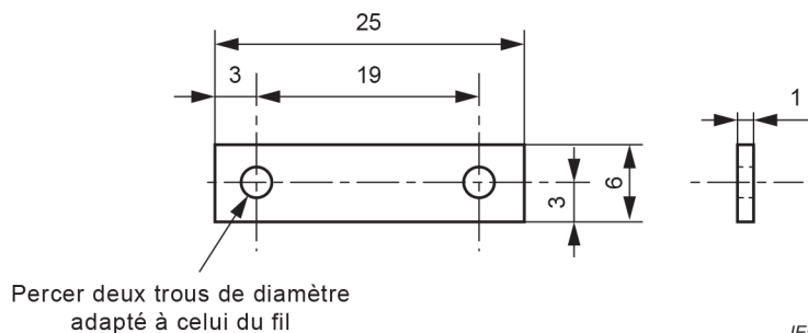
Figure 2 –Séparateur
