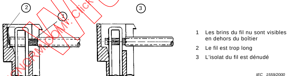
Figure 18 – Connexions CAD défectueuses; détérioration physique du fil câblé
