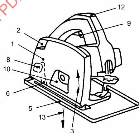
Figure 102 – Scie circulaire à protecteur pendulaire intérieur
