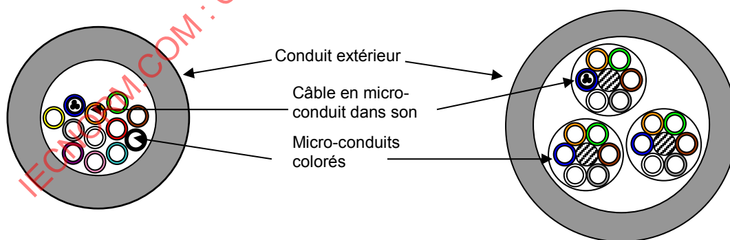
Figure A.1 – Câbles à fibres optiques en micro-conduit (non à l'échelle)
