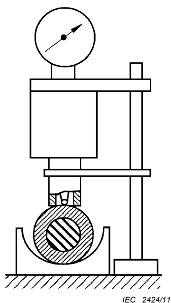
Figure H.2a – Éprouvette dans une goulotte
