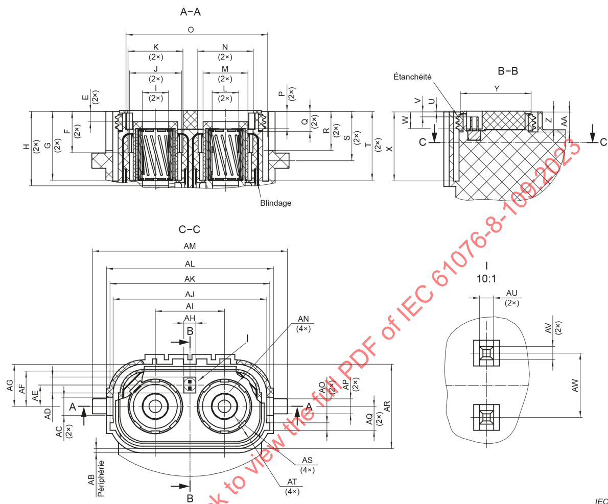
Figure 3 – Fiche
