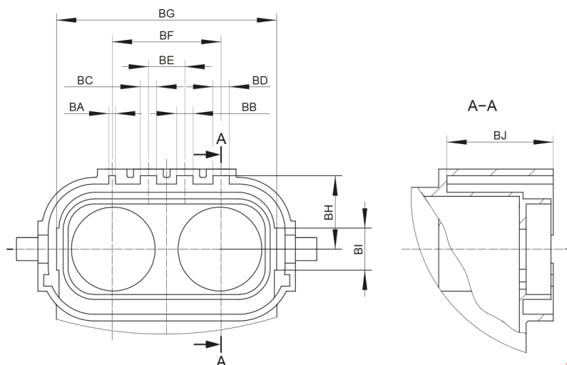
Figure 4 – Détrompages des fiches
