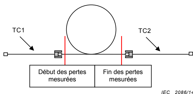
Figure 4 – Configuration B – Début et fin de pertes mesurées dans la méthode d'essai de référence
