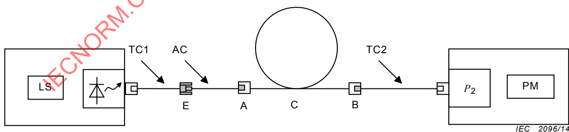
Figure C.2 – Mesure d'essai à deux cordons
