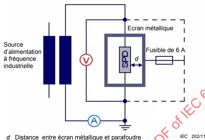
Figure 1 – Montage d'essai de l'écran métallique
