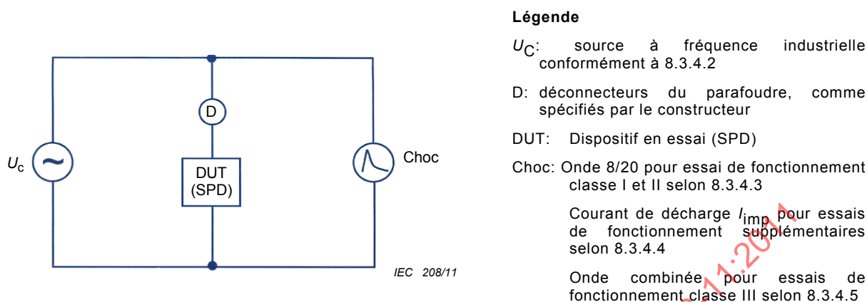
Figure 7 – Schéma du circuit d'essai de fonctionnement
