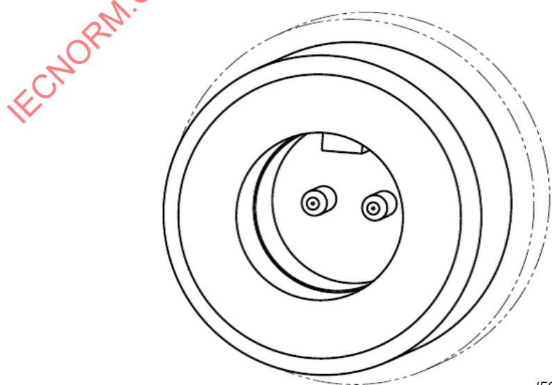
Figure 3 – Connecteur femelle à deux voies (vue isométrique)
