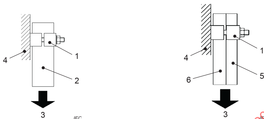
a) Essai de tenue à la charge axiale sur une bride de câbles recevant un câble
