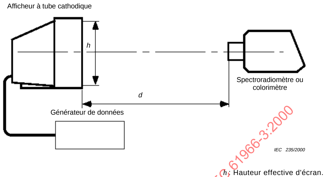
Figure 1 – Disposition de l'équipement pour mesures sans contact
