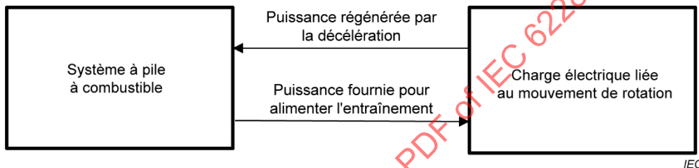
Figure 4 – Circulation de l'énergie pour la puissance régénérée et la puissance fournie
