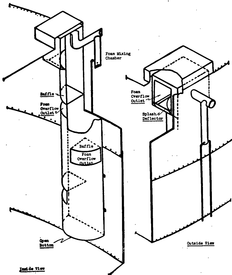
Fig. A-302C. Foam Chute.
