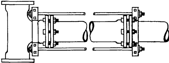
FIG. 96-14. TEE ANCHOR
