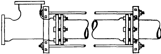
FIG. 96-13. TEE ANCHOR
