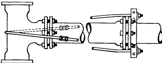
FIG. 96-12. TEE ANCHOR
